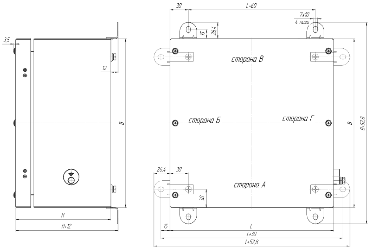
Рисунок А.1 – Габаритно – монтажный чертеж исполнений КВУ-10
